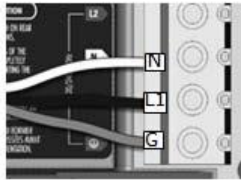
120 V (*3 wires)
