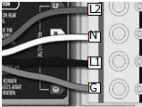
240 V (4 wires)
